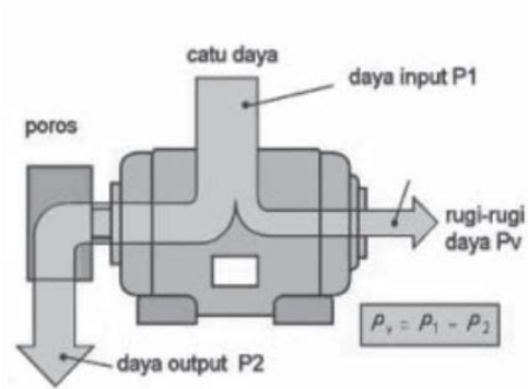
Gambar-2. Motor Induksi.
