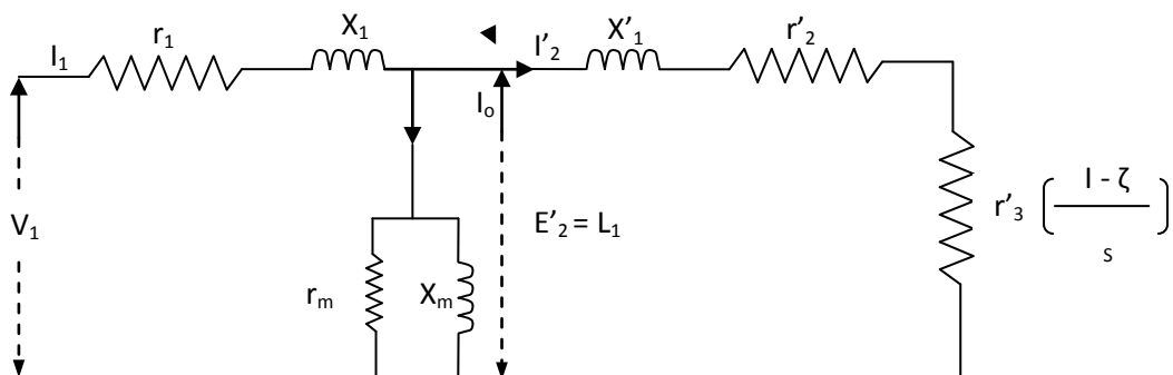
Gambar-2. Rangkaian Ekvaleen Motor Induksi Perfasa
