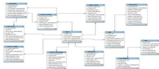
Gambar 3. ERD
