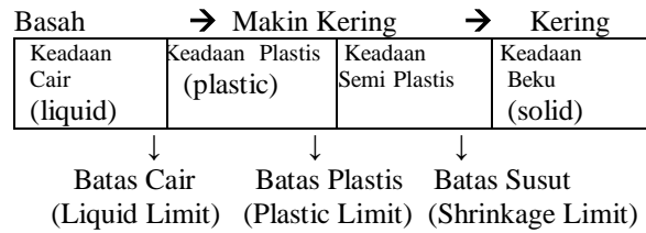
Gambar 2. Skema Batas-batas Atterberg
